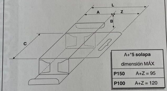
4 — cierre a encastre con solapas pares + 5° solapa
