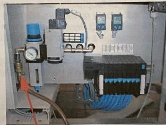
Embrayage rapide
